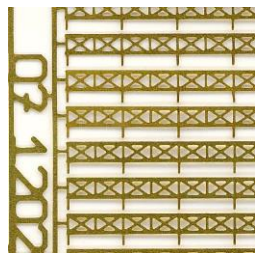
07-1202 20 St. H2,8 L.187 mm, 51 Felder
