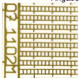
07-1102 24 St. H2,3 L.188 mm
